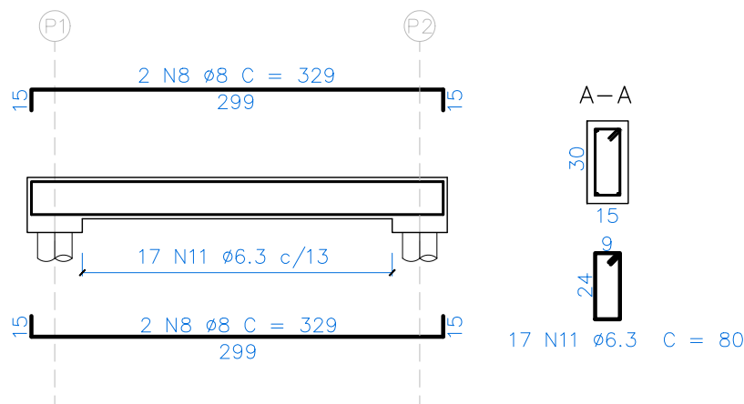
VIGA BALDRAME VB01 (15 x 30)
