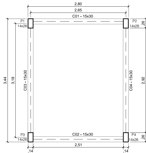
ESTRUTURA FORMA DA COBERTURA (NÍVEL 260cm) ESC: 1:50
