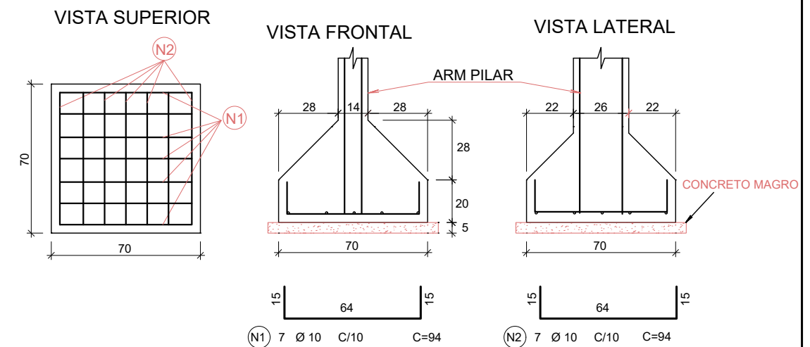
ESTRUTURA DETALHES DAS SAPATAS ESC: 1:25
