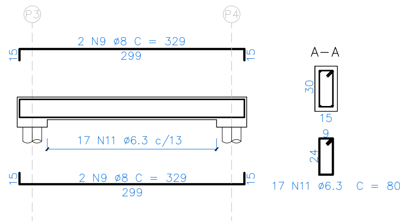
VIGA BALDRAME VB02 (15 x 30)
