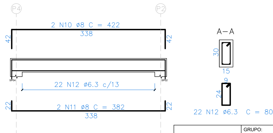
VIGA BALDRAME VB04 (15 x 30)
